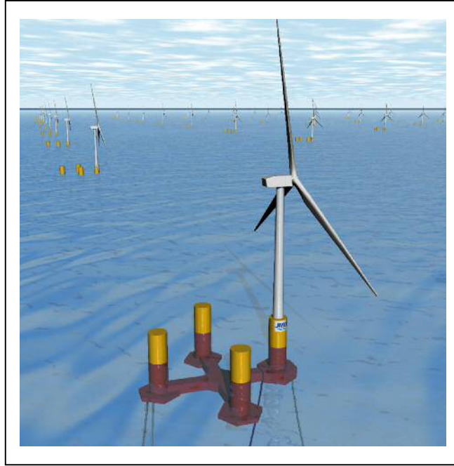
JMU 独自開発、大型風車対応のセミサブ型洋上風車浮体イメージ
